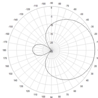
Horizontal beamwidth
